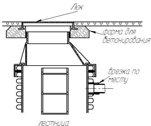
Схема сборки колодца и установки люка
